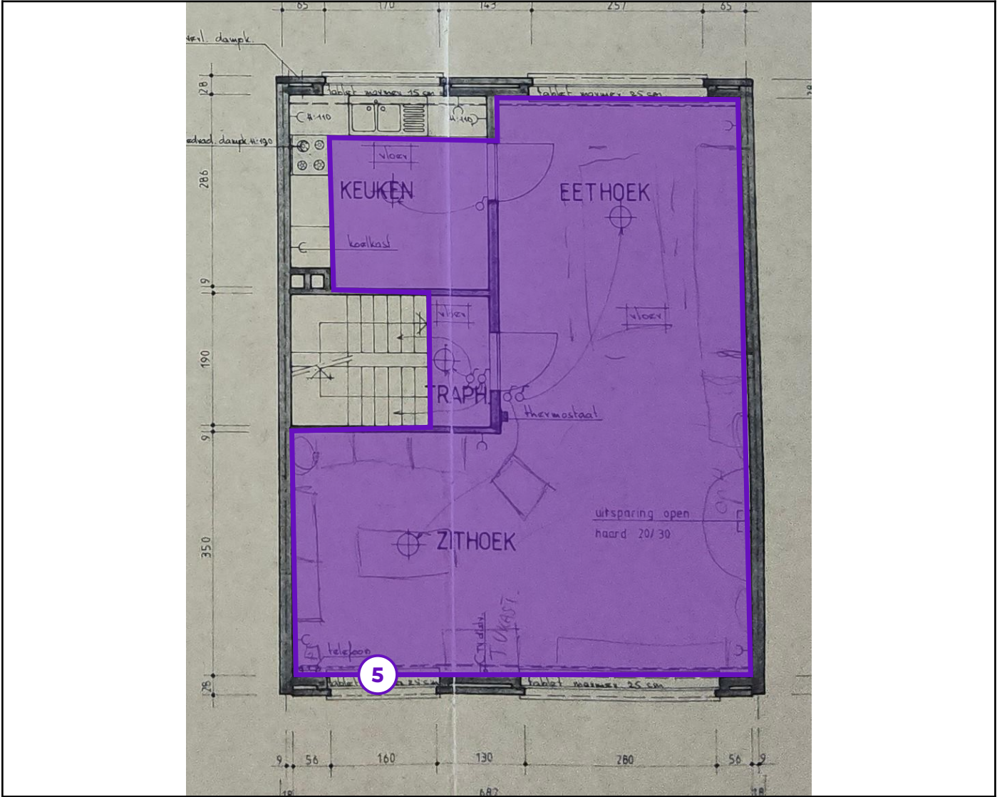
Legende van plan 1.7: Eerste verdieping
