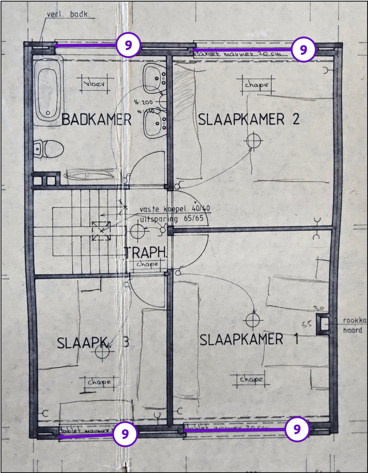
Legende van plan 1.10: Tweede verdieping
